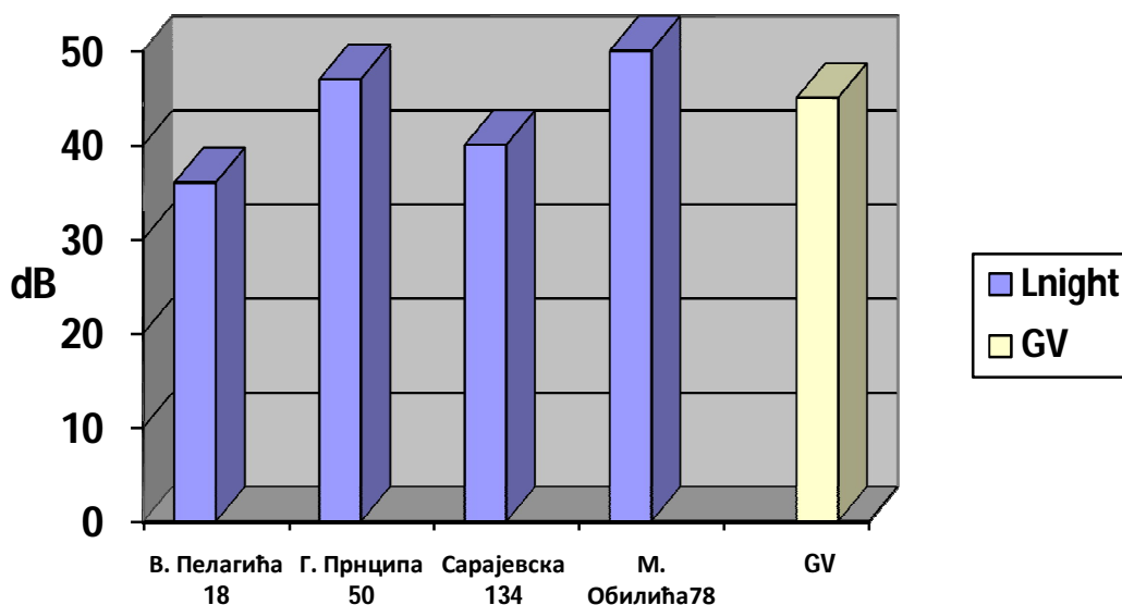
Графикон 7. Ноћни ниво буке и гранична вредност индикатора буке за ноћ у dB(A). Мерна места у зони становања: В. Пелагића 18, Г. Прнципа 50, Сарајевска 134 и М. Обилића 78, Вршац. Јесења сезона 2015.
